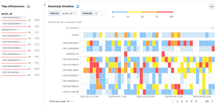
Рисунок 7. Приклад результату виявлення аномалій у переглядах для окремих Telegram каналів
