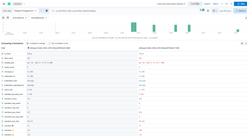
Рисунок 3. Приклад порівняння документів
