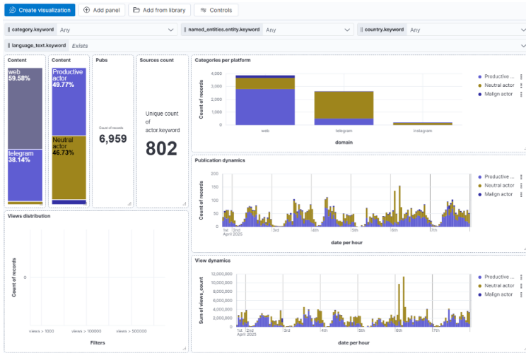
Рисунок 5. Приклад дашборду в інтерфейсі Dashboards
