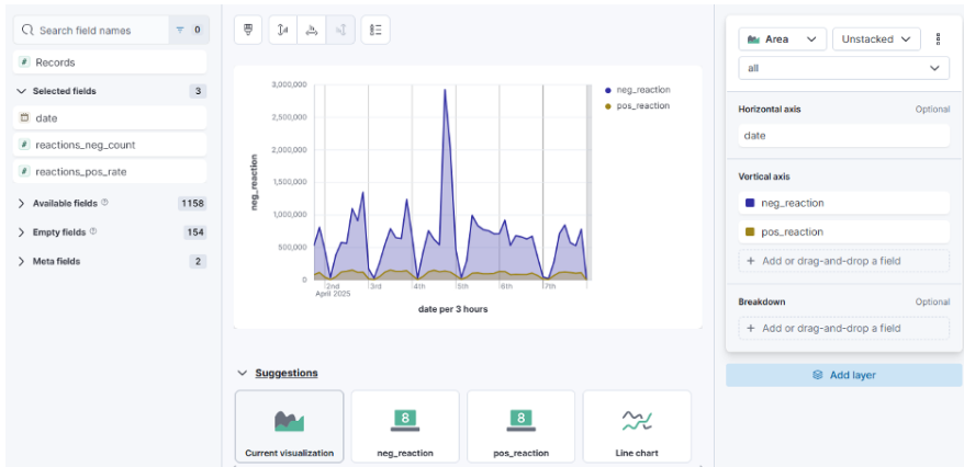
Рисунок 4. Приклад візуалізації в інтерфейсі Lens
